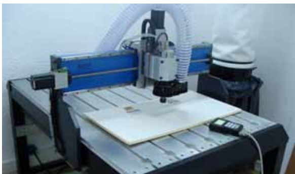
Router CNC para fabricación de modelos sólidos
